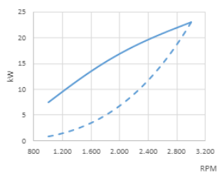
Effektkurva (ISO 3046/1)
